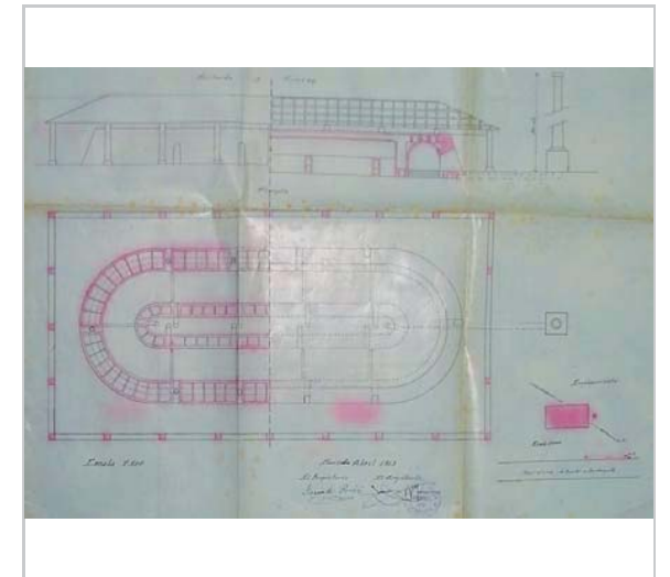
Plànol del projecte. Joan B. Serra 1923 Arxiu Municipal de Montcada i Reixac
